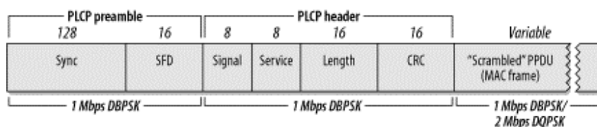
Figure 10-23. DS PLCP framing
